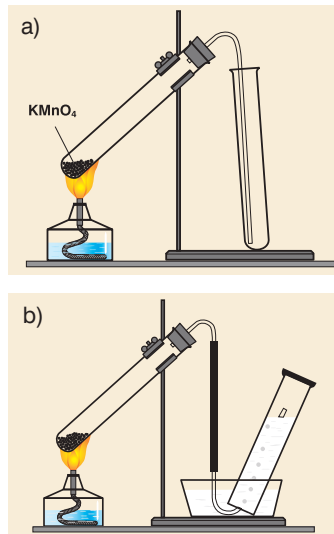
Fig. 3.8. Captarea oxigenului prin dezlocuirea a) aerului; b) apei.
