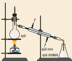
Fig. 5.33. Instalație pentru distilarea apei în laborator.
