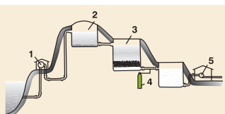
Fig. 5.31. Schema stației de epurare a apei: 1 – pompă; 2 – bazin de decantare; 3 – filtru; 4 – dispozitiv pentru clorurarea apei; 5 – pomparea apei spre consumator.
