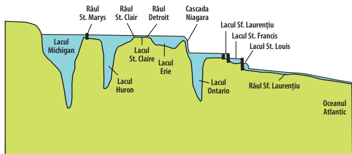
Fig. 1.41. Profil de la Marile Lacuri până la Oceanul Atlantic
