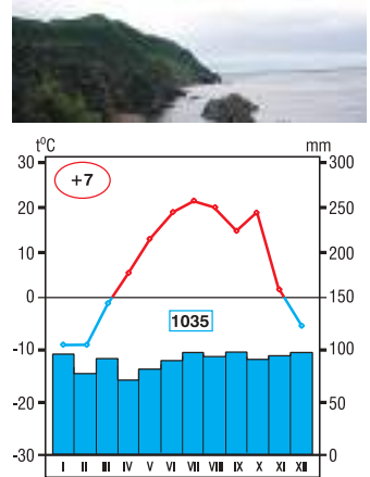
Fig. 1.31. Climogramă, or. Mont-réal, 45°30' lat. N (Canada)
