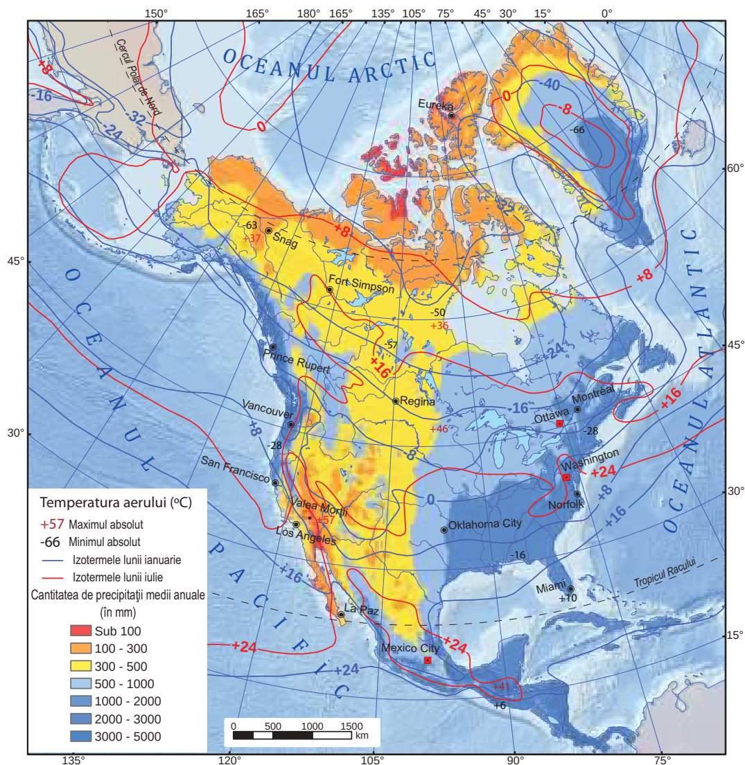
Fig. 1.23. Distribuția temperaturii aerului și a precipitațiilor atmosferice în America de Nord
