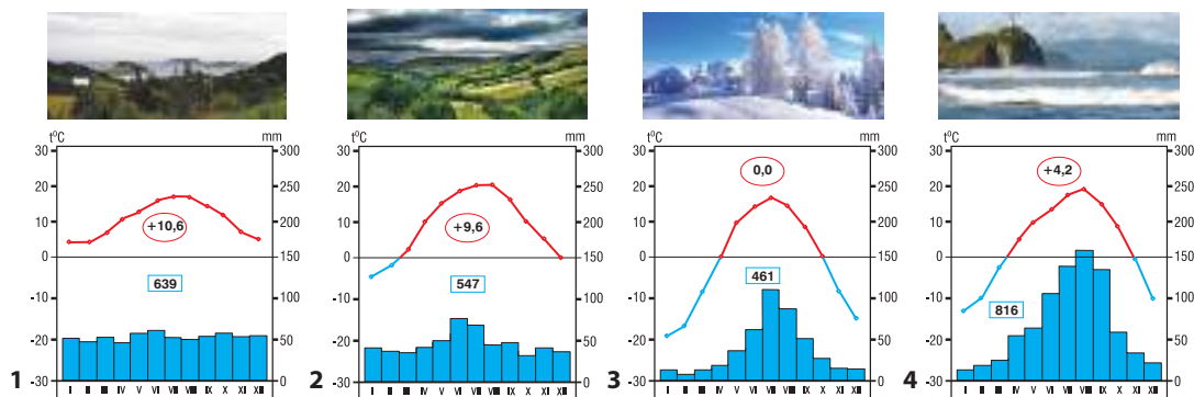
Fig. 2.65. Climograme (zona temperată)
