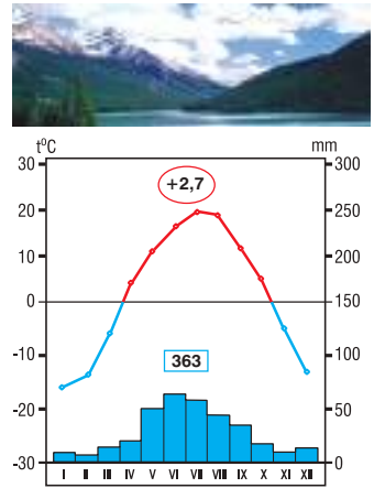
Fig. 1.30. Climogramă, or. Regi-na, 50°27' lat. N (Canada)
