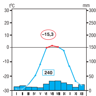
Fig. 2.63. Climogramă, capul Celiuskin (Rusia), 77°43' lat. N
