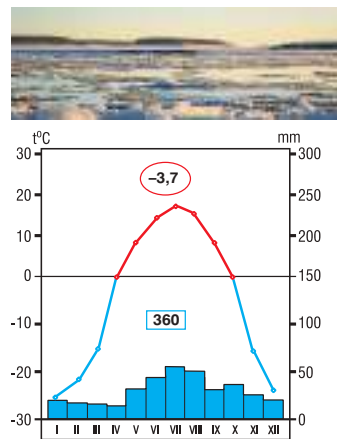
Fig. 1.32. Climogramă, or. Fort Simpson, 61°51' lat. N (Canada)
