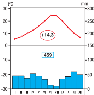
Fig. 2.51. Climogramă, or. Madrid (Spania), 40°24' lat. N
