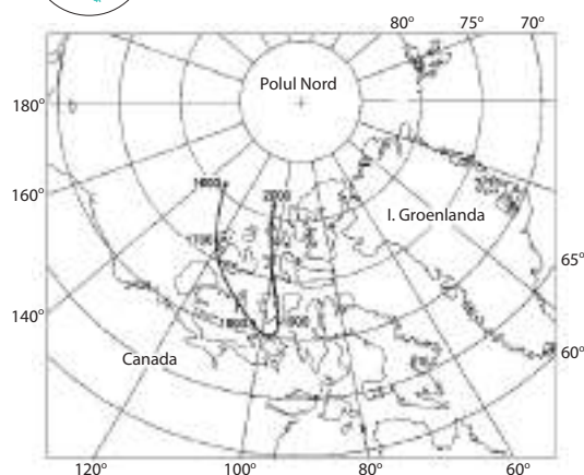
Fig. 1.4. Deplasarea Polului Nord Magnetic între anii 1600-2000
